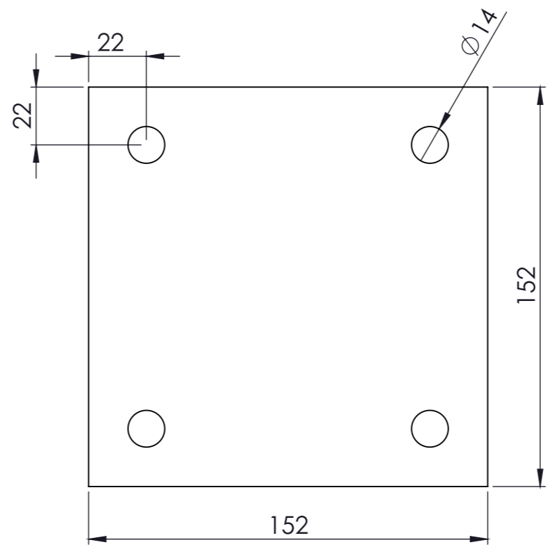
VISTA INFERIOR
