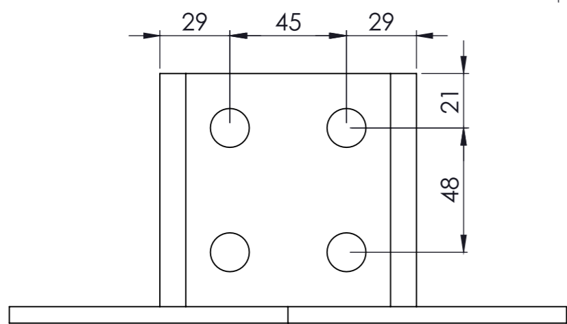
VISTA POSTERIOR
