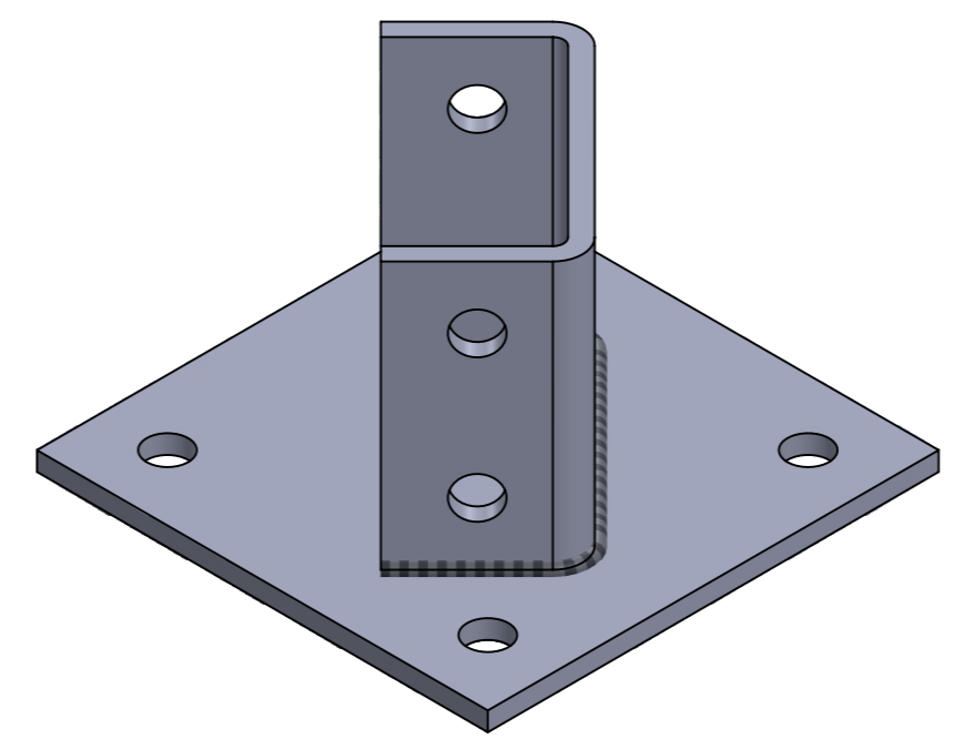
VISTA ISOMETRICA
